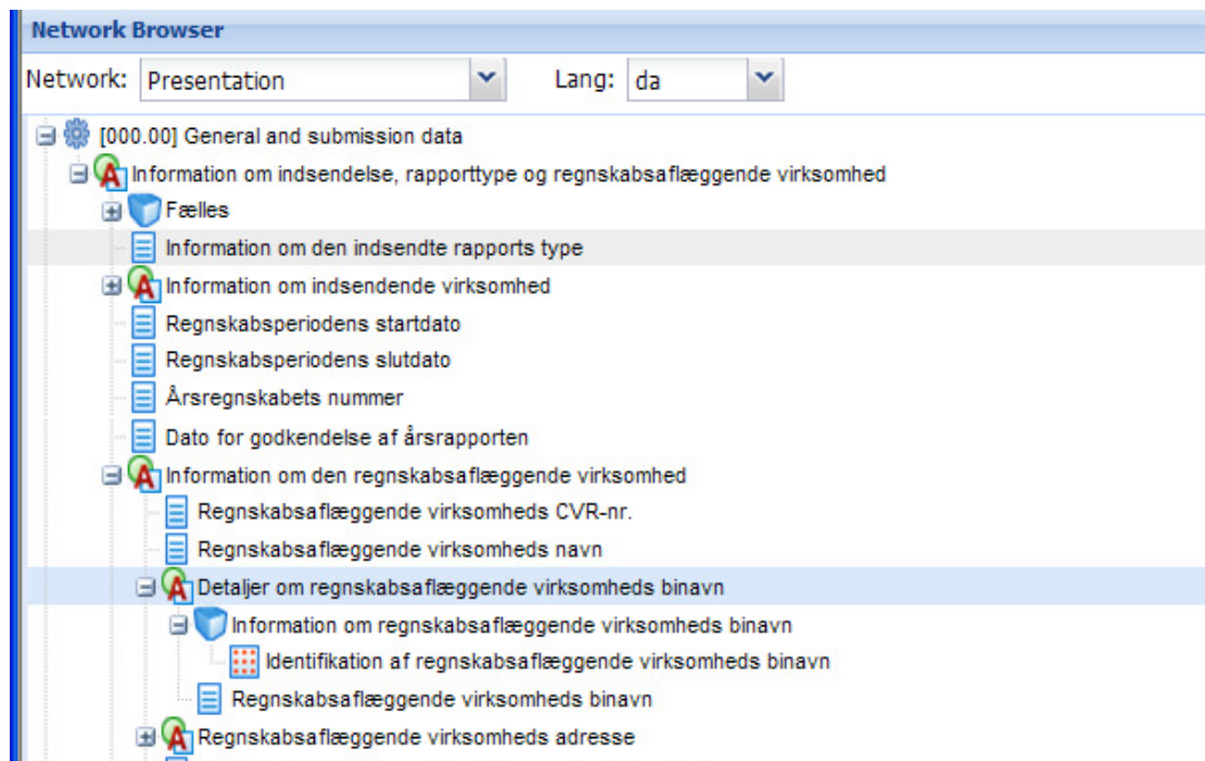
Figur 2: Visning af virksomhedens eventuelle binavne
