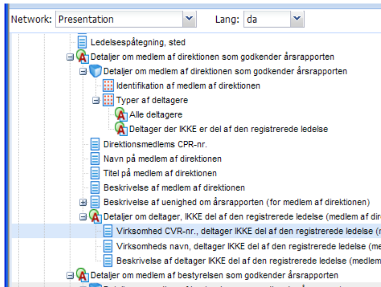
Figur 5: Visning af detaljer om deltager i ledelsen, som ikke er en del af den registrerede ledelse
